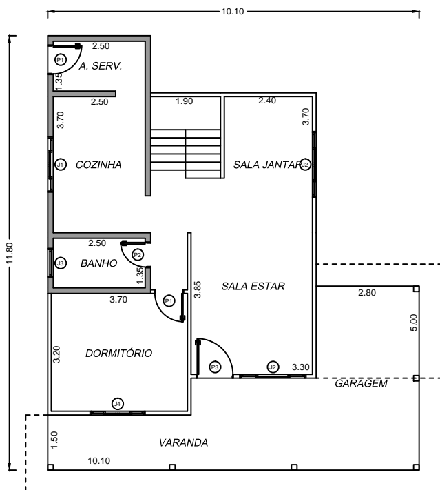
PAVIMENTO TÉRREO: 93,16 M 2
