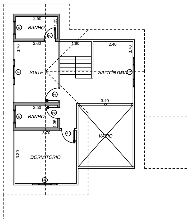
PAVIMENTO SUPERIOR: 64,81 M 2
