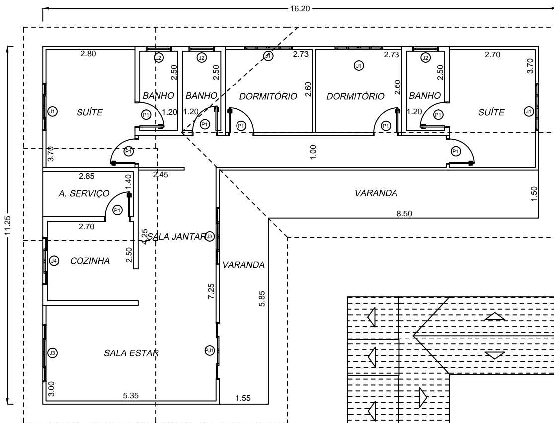
PAVIMENTO TÉRREO: 125,77 M 2
